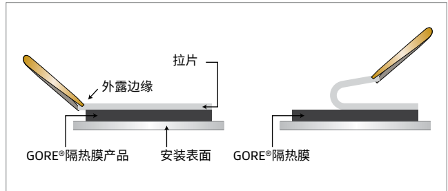
图5：取下拉片
