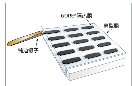
图2：卷起离型膜
